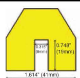
Edge Guard Type BB
