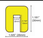
Edge Guard Type G
